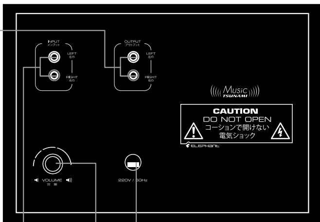
Subwoofer (back view) サブウーファー (背面図)
